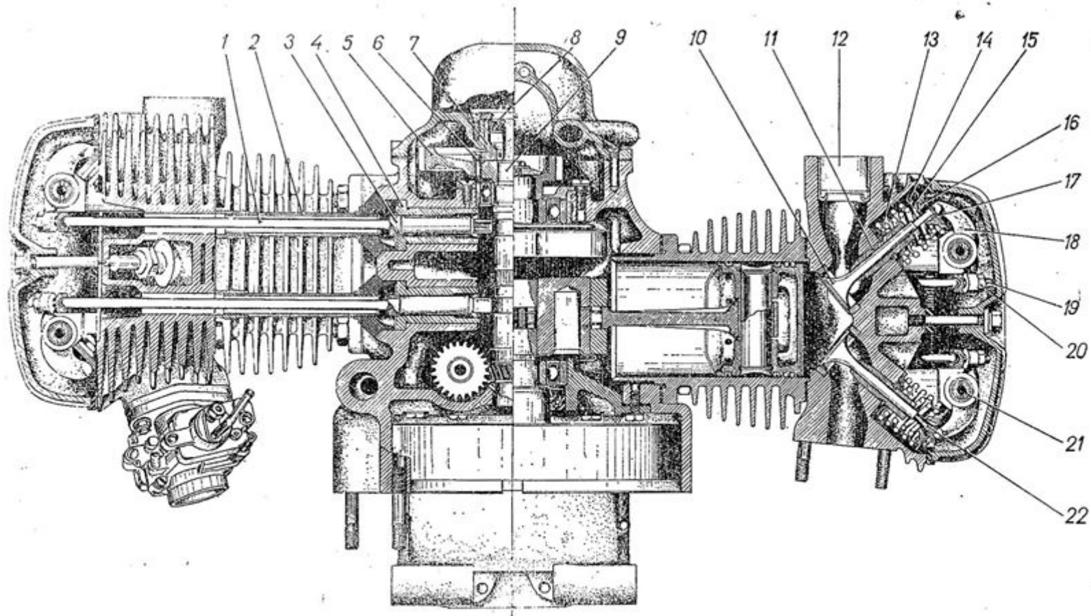
Рис. 6. Механизм газораспределения двигателя:
