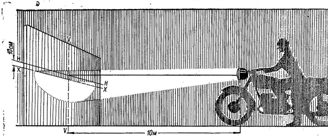
Рис. 27. Схема проверки установки фары
