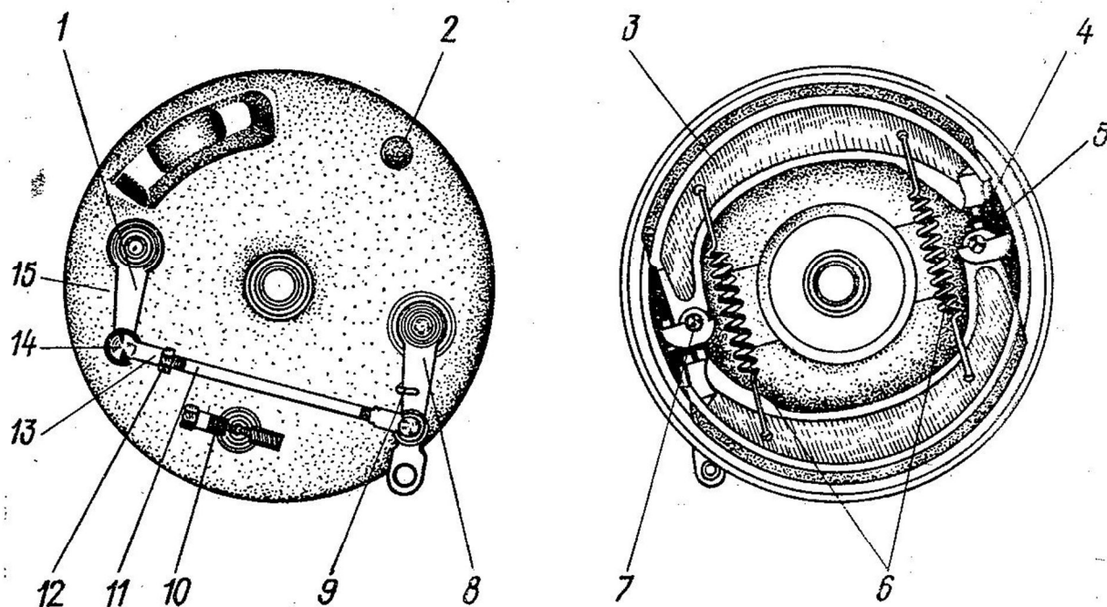
Рис. 24. Тормоз переднего колеса:
