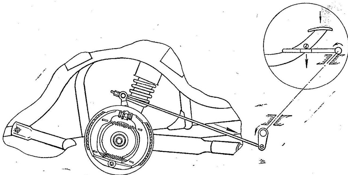
Рис. 25. Тормоз колеса коляски
