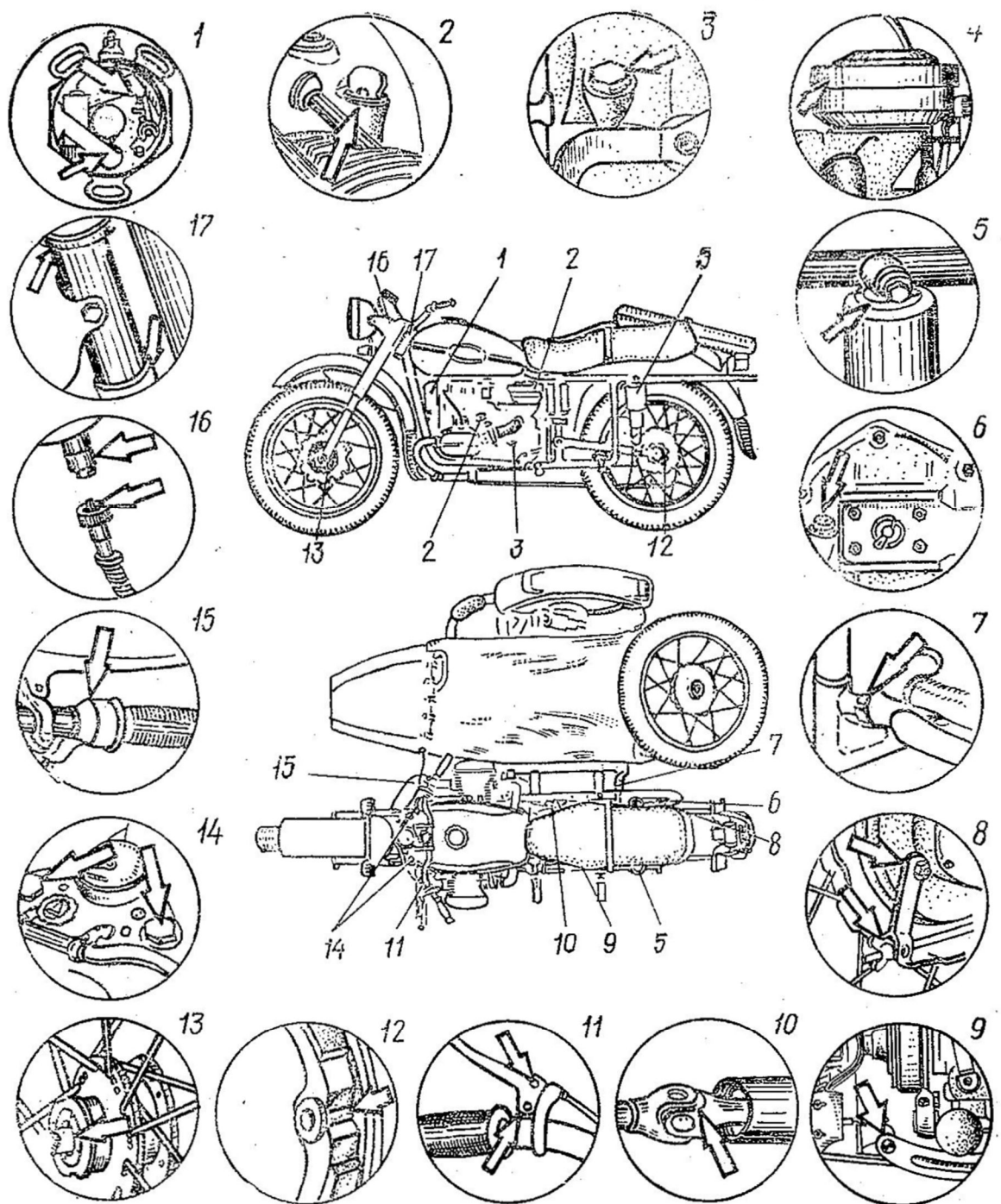
Рис. 32. Химмотологическая карта:
