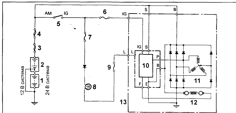
Схема системы зарядки (Дуна, Toyota). 1 - аккумуляторная батарея, 2 - аккумуляторная батарея, 3 - главная плавкая вставка (2,0L), 4 - плавкая вставка "AM1" (50A) (24В система) или "AM1" (60A) (12В система), 5 - замок зажигания, 6 - предохранитель "GAUGE ENGINE" (10A) (модификация для Европы (Wide Cab)) или "ENGINE" (7,5A) (остальные модификации), 7 - предохранитель "GAUGE" (10A) (модификация для Европы (Wide Cab)) или (7,5A) (остальные), 8 - контрольная лампа зарядки аккумуляторной батареи, 9 - предохранитель "CHARGE" (7,5A), 10 - регулятор напряжения, 11 - обмотка статора, 12 - обмотка ротора, 13 - генератор.
