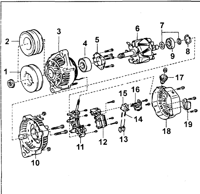
Генератор (12В система) (3В, 14В, 15В-Ф, 15В-ФТ, модели выпуска с 1995 года). 1 - шкив (одинарный ремень), 2 - шкив (двойной ремень), 3 - крышка генератора (в сборе со статором), 4 - передний подшипник, 5 - держатель подшипника, 6 - ротор, 7 - крышка подшипника, 8 - шайба генератора, 9 - задний подшипник, 10 - корпус выпрямительного блока, 11 - выпрямительный блок, 12 - регулятор напряжения, 13 - щетка, 14 - пружина, 15 - щеткодержатель, 16 - крышка щеткодержателя, 17 - изолятор вывода, 18 - крышка генератора со стороны выпрямительного блока, 19 - зажим проводки.
