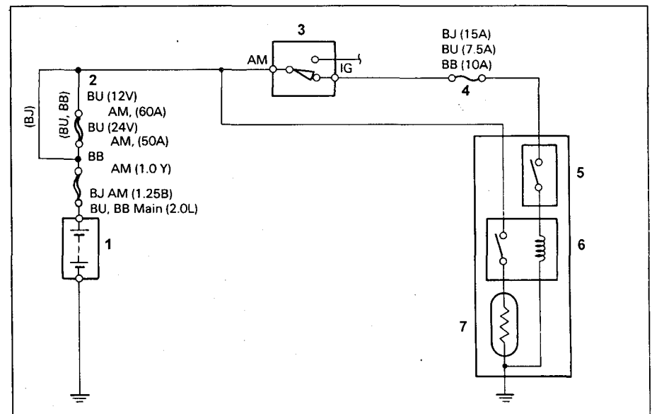
Электросхема системы подогрева топлива. 1 - аккумуляторная батарея, 2 - плавкая вставка, 3 - замок зажигания, 4 - предохранитель, 5 - выключатель, 6 - реле нагревателя, 7 - нагреватель.
