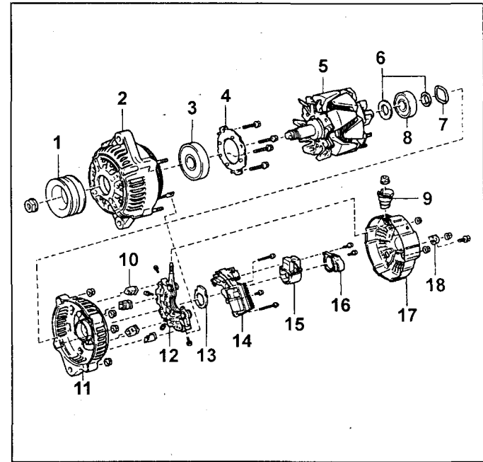
Генератор (24В система) (3В, 14В, 15В-Ф, 15В-ФТ, модель Coaster выпуска с мая 1995 года). 1 - шкив, 2 - крышка генератора (в сборе со статором), 3 - передний подшипник, 4 - держатель подшипника, 5 - ротор, 6 - крышка подшипника, 7 - шайба генератора, 8 - задний подшипник, 9 - изолятор вывода, 10 - резиновый изолятор, 11 - корпус выпрямительного блока, 12 - выпрямительный блок, 13 - уплотнительная пластина, 14 - регулятор напряжения, 15 - щеткодержатель, 16 - крышка щеткодержателя, 17 - крышка генератора со стороны выпрямительного блока, 18 - вывод.
