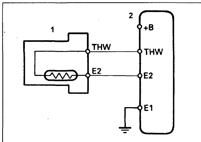
1 - датчик температуры охлаждающей жидкости, 2 - электронный блок управления.
