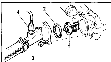
Снятие термостата 4A-GE.
