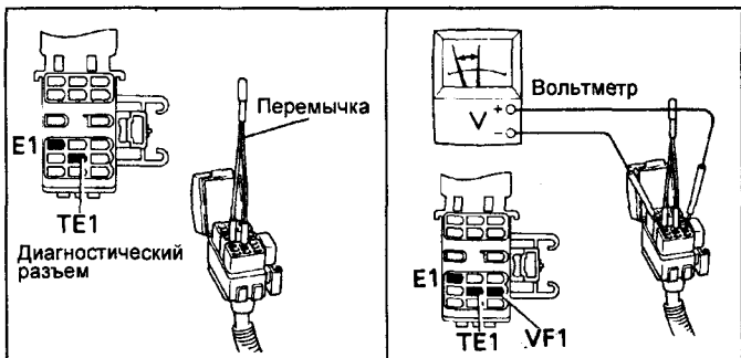
Схемы подключения кислородного датчика и/или датчика обедненного состава смеси (5A-FE). 1 - диагностический разъем, 2 - кислородный датчик, 3 - электронный блок управления.
