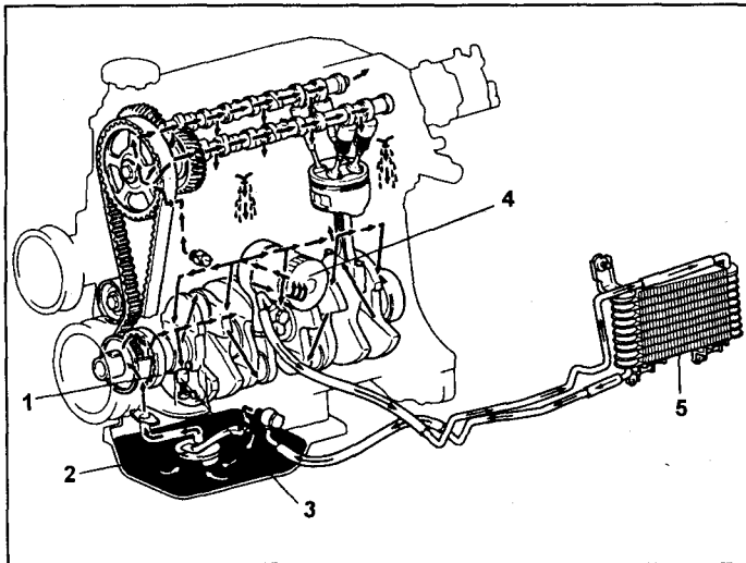
Схема расположения элементов системы смазки двигателей 4A-FE, 5A-FE и 7A-FE. 1 - масляный насос, 2 - маслоприемник, 3 - редукционный клапан, 4 - масляный фильтр, 5 - масляный радиатор.
