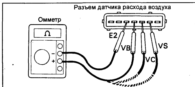
Схема подключения омметра к выводам расходомера воздуха
