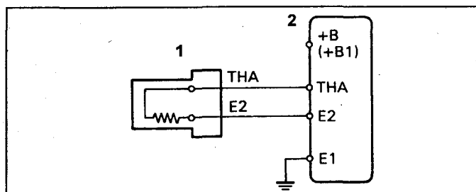
Двигатели без расходомера воздуха. 1 - датчик температуры воздуха на впуске, 2 - электронный блок управления.
