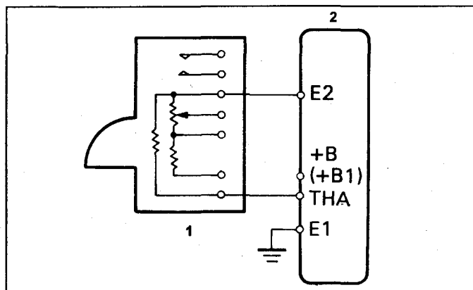
Двигатели с расходомером воздуха. 1 - датчик температуры воздуха на впуске, встроенный в расходомер воздуха, 2 - электронный блок управления.
