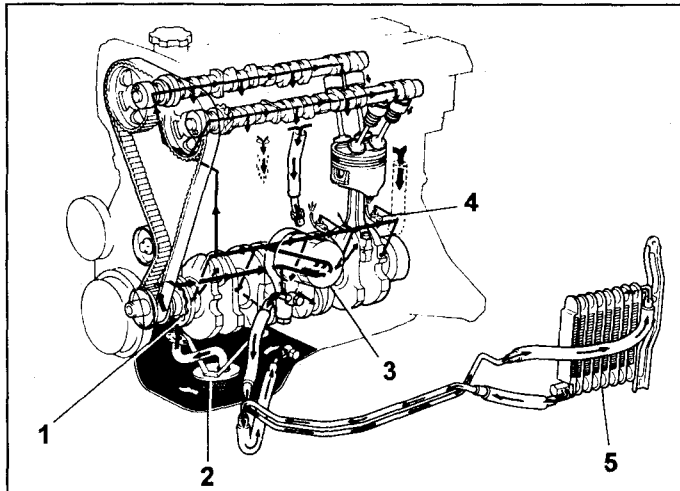
Схема расположения элементов системы смазки двигателя 4A-GE. 1 - масляный насос, 2 - маслоприемник, 3 - масляный фильтр, 4 - форсунка для подачи масла на днище поршня и стенки цилиндров, 5 - масляный радиатор.
