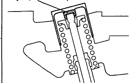
Регулировочная прокладка
