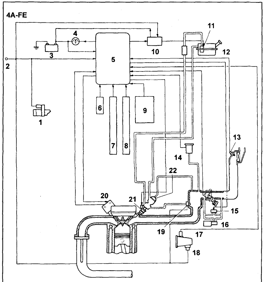
Схема системы впрыска топлива двигателей 4A-FE для моделей 2WD (AE92, AE95, AT171 и AT180) вариант без системы рециркуляции отработавших газов. 1 - стартер, 2 - замок зажигания, 3 - аккумуляторная батарея, 4 - контрольная лампа "CHECK", 5 - электронный блок управления, 6 - компрессор кондиционера, 7 - переменный резистор, 8 - датчик частоты вращения, 9 - датчик положения дроссельной заслонки, 10 - реле-выключатель топливного насоса, 11 - топливный бак, 12 - датчик температуры воздуха на впуске, 13 - датчик абсолютного давления во впускном коллекторе, 14 - клапан системы управления частотой вращения холостого хода, 15 - клапан системы управления подачей воздуха, 16 - датчик температуры охлаждающей жидкости, 17 - термовременное реле форсунки холодного пуска, 18 - форсунка холодного пуска, 19 - объединенный блок зажигания, 20 - форсунка, 21 - регулятор давления топлива.
