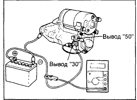
Стартер с обычным редуктором.
