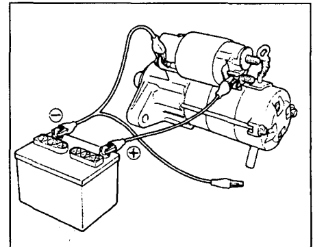
Стартер с обычным редуктором.
