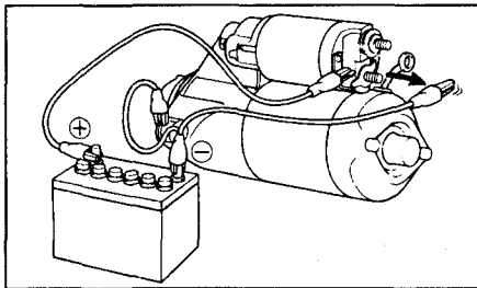
Стартер с планетарным редуктором.
