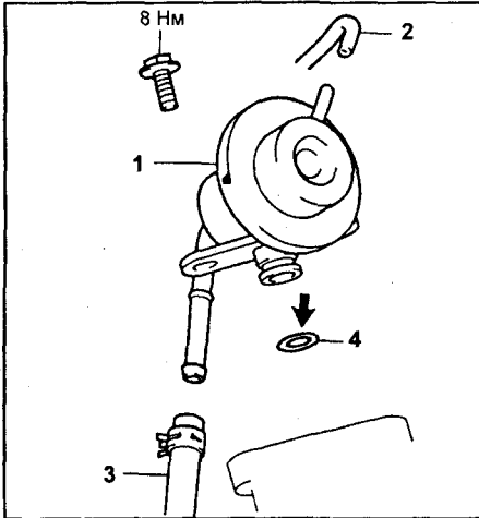
Регулятор давления топлива (4A-GE для AE111). 1 - регулятор, 2 - вакуумный шланг, 3 - шланг возврата топлива, 4 - кольцевое уплотнение.
