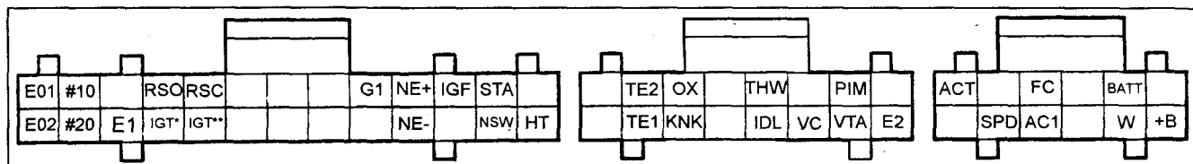
Выходы электронного блока управления (4A-FE (AE111), 5A-FE (AE110), 7A-FE (AE115)).
