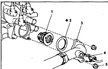
Снятие термостата 4A-FE, 5A-FE и 7A-FE.
