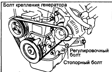
4А-ФЕ, 5А-ФЕ и 7А-ФЕ.
