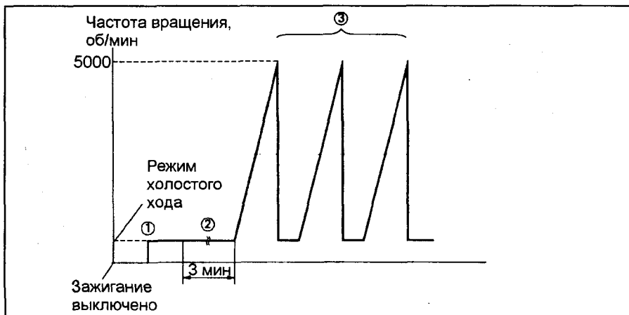
Код № 52 - Датчик детонации.
