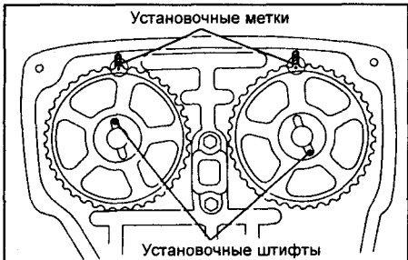
Установочные штифты
