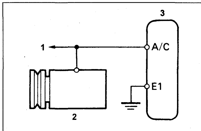
1 - усилитель кондиционера, 2 - компрессор кондиционера, 3 - электронный блок управления.
