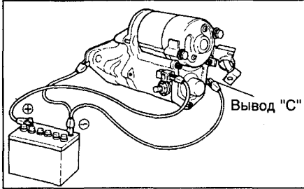
Стартер с обычным редуктором.
