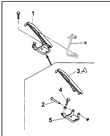
Педаль акселератора. 1 - педаль акселератора в сборе, 2 - штифт, 3 - педаль акселератора, 4 - стопорный болт, 5 - кронштейн, ● - рычаг акселератора.
