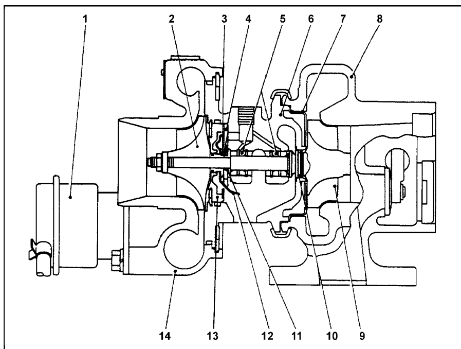
Устройство турбокомпрессора. 1 - привод клапана перепуска ОГ, 2 - колесо компрессора, 3 - вал компрессора, 4 - упорный подшипник, 5 - подшипник, 6 - корпус подшипников, 7 - задняя пластина турбины, 8 - корпус турбокомпрессора, 9 - вал и колесо турбины, 10, 11 - кольцевое уплотнение, 12 - маслоотражатель, 13 - вкладыш, 14 - крышка компрессора.
