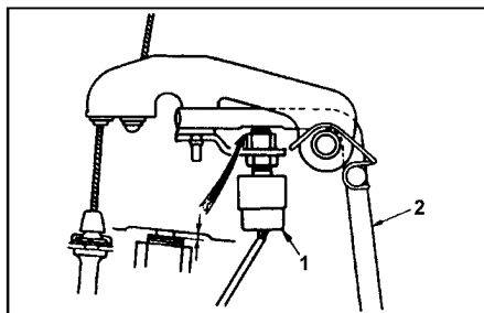
Hyundai. 1 - концевой выключатель, 2 - рычаг педали акселератора.
