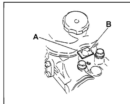
4D33, 4D34-T4, 4D35, D4AK, D4AF, D4AE. А - место установки форсунки, В - ветошь.
