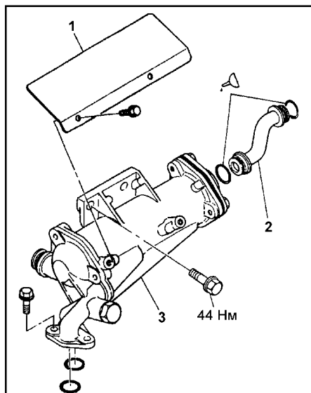
Снятие и установка маслоохладителя (D4AF, D4AK, D4AE). 1 - теплозащитный экран, 2 - трубка охлаждающей жидкости, 3 - маслоохладитель.
