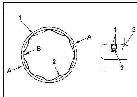
1 - уплотнительное кольцо, 2 - расширитель, 3 - соединительное кольцо.
