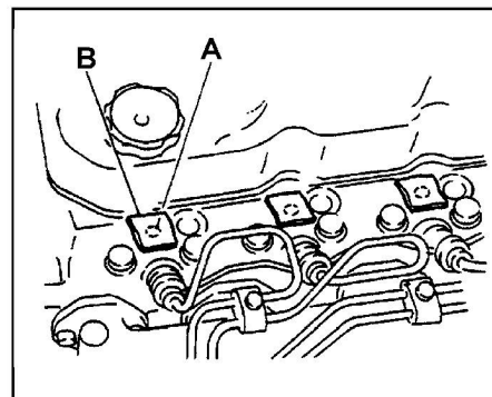
4D36. А - место установки свечи накалывания, В - ветошь.
