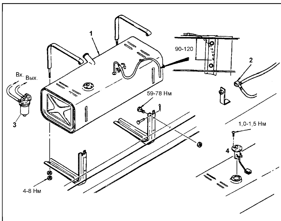
Снятие и установка топливного бака на 100 литров (Hyundai). 1 - топливный бак, 2 - клапан, 3 - водоотстойник, 4 - датчик уровня топлива.
