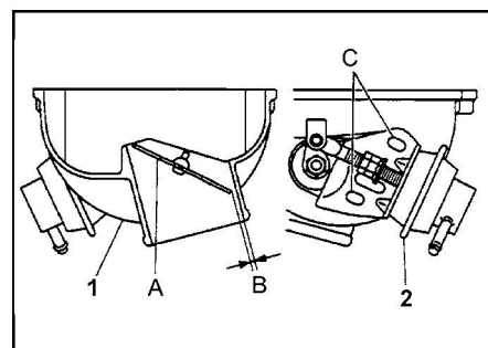
4D35. 1 - нижняя часть впускного коллектора, 2 - привод, А - дроссельная заслонка, В - зазор, С - регулировочное отверстие кронштейна.
