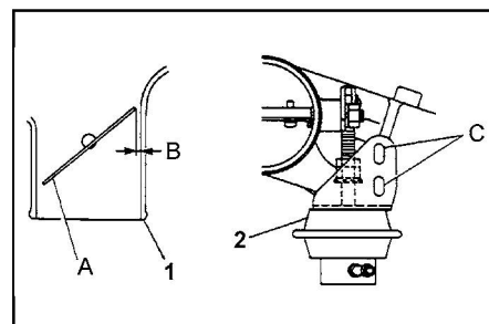
4D33, 4D34-T4, 4D36. 1 - нижняя часть впускного коллектора, 2 - привод, А - дроссельная заслонка, В - зазор, С - регулировочное отверстие кронштейна.
