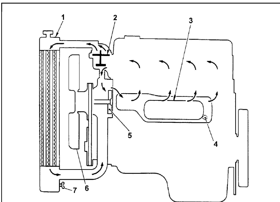
Схема системы охлаждения двигателя (MCC Canter). 1 - радиатор, 2 - термостат, 3 - маслоохладитель, 4 - сливная пробка блока цилиндров, 5 - насос охлаждающей жидкости, 6 - вентилятор системы охлаждения, 7 - сливная пробка радиатора.
