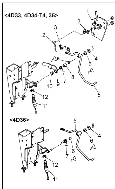
Рычаг педали акселератора (MMC Canter). 1* - датчик положения педали акселератора, 2* - шток датчика, 3* - втулка, 4 - шайба, 5 - рычаг педали акселератора, 6 - втулка, 7 - пружина, 8 - направляющая втулка, 9 - рычаг, 10 - втулка, 11 - концевой выключатель (на педали акселератора), 12 - гайка, ● - модели с АКПП, с системой изменения усилия на рулевом колесе в зависимости от скорости движения.
