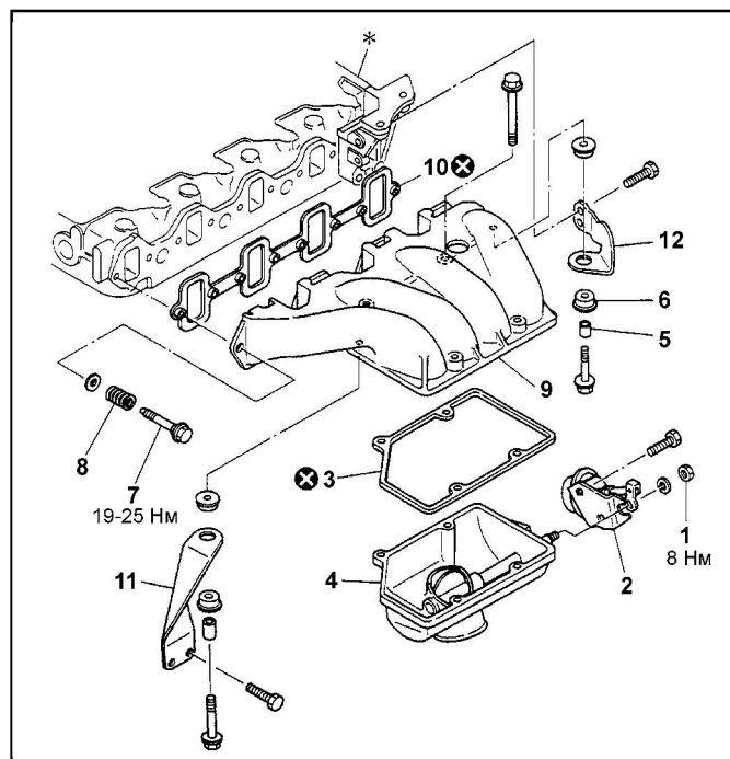
Снятие и установка впускного коллектора (4D35) (модели выпуска до 1995 года). 1 - гайка, 2 - привод, 3 - прокладка, 4 - нижняя часть впускного коллектора, 5 - проставка, 6 - резиновая подушка, 7 - болт, 8 - пружина, 9 - впускной коллектор, 10 - прокладка, 11, 12 - кронштейн, * - головка блока цилиндров.
