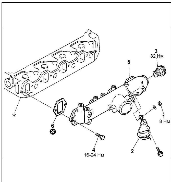
Снятие и установка впускного коллектора (4D33, 4D34-T4, 4D36) (модели выпуска до 1995 года). 1 - гайка, 2 - привод, 3 - клапан перепуска наддувочного воздуха, 4 - болт, 5 - впускной коллектор, 6 - прокладка, * - головка блока цилиндров.
