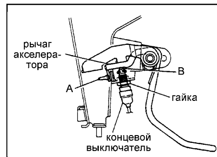
Hyundai. 1 - концевой выключатель, 2 - рычаг педали акселератора.
