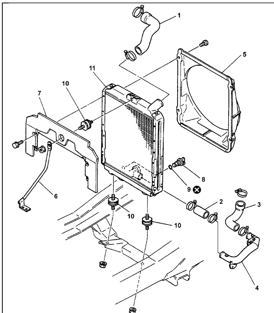
Снятие и установка радиатора (4D33, 4D34-T4, 4D35, 4D36, модели выпуска после 1995 года). 1 - впускной шланг радиатора, 2, 3 - выпускной шланг радиатора, 4 - трубка, 5 - диффузор вентилятора, 6 - стойка радиатора, 7 - экран, 8 - сливная пробка радиатора, 9 - кольцевое уплотнение, 10 - опора, 11 - радиатор.
