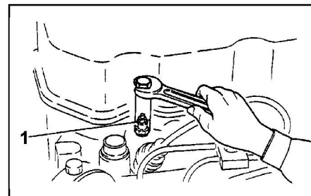
1 - свеча накалывания.
