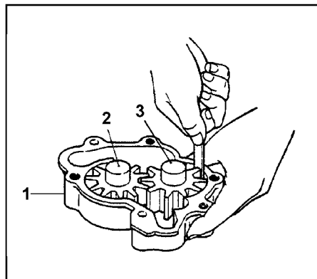
1 - корпус масляного насоса, 2 - ведущий ротор, 3 - ведомый ротор.
