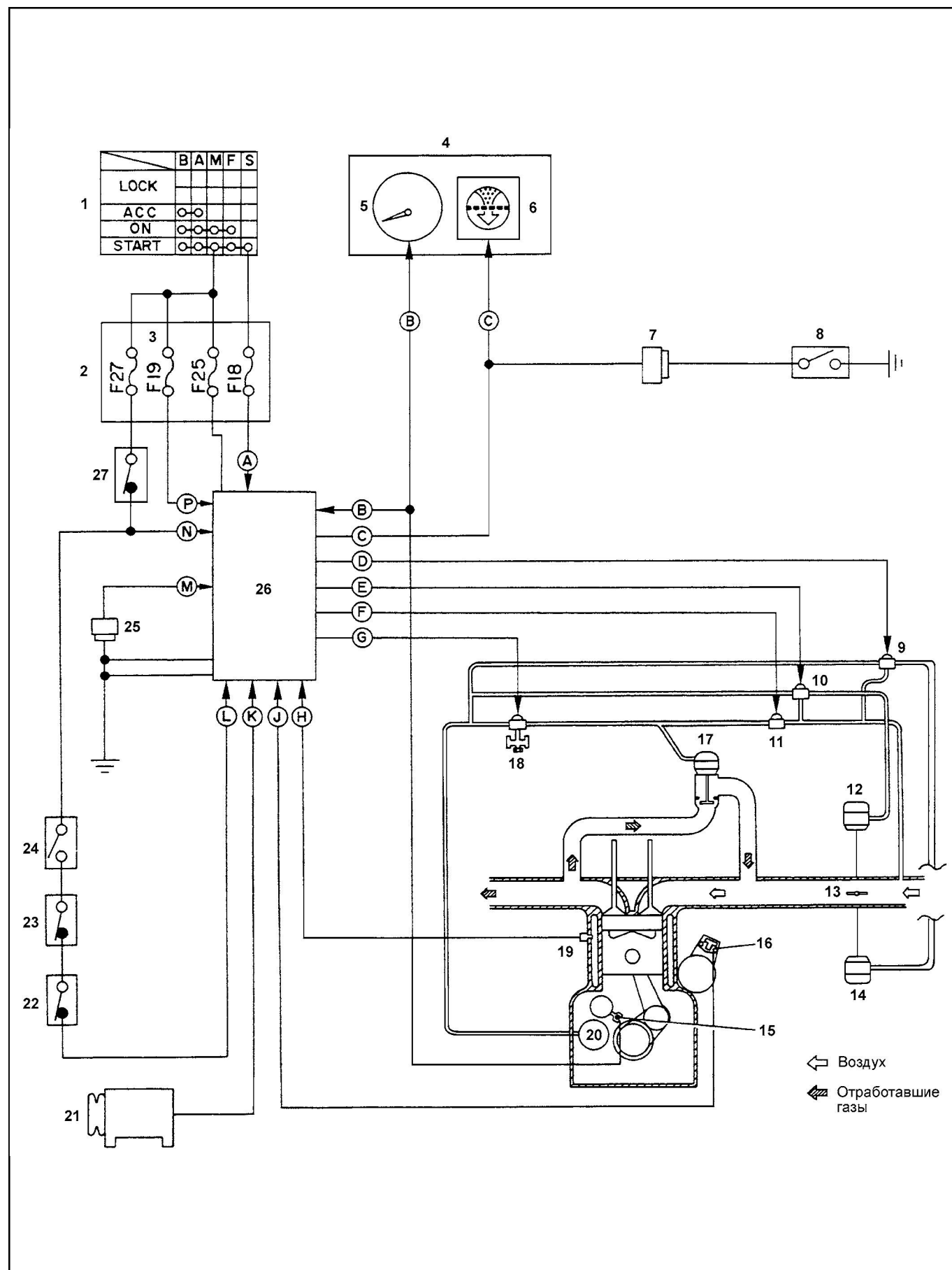
Система рециркуляции отработавших газов (модели выпуска после 1997 года).
