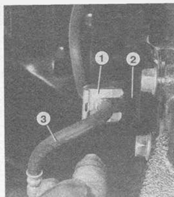
Демонтаж тормозного шланга
