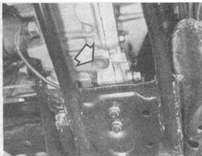
Резьбовая пробка отверстия (стрелка) для слива масла из коробки передач находится в выемке сзади (в направлении движения).
