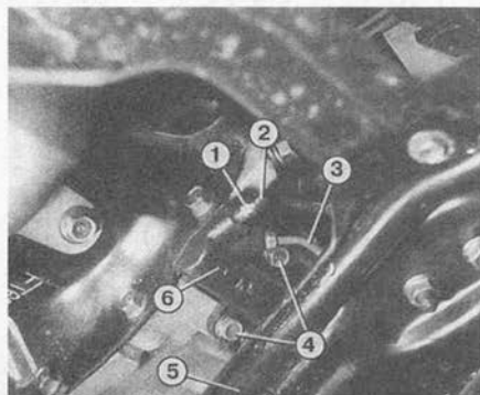
Вид с нижней стороны автомобиля на главный цилиндр сцепления на коробке передач. Цифрами обозначены следующие детали:
