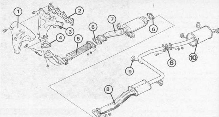
Детали выхлопной системы: 1 – теплоизолирующий щиток; 2 – прокладка выпускного коллектора; 3 – выпускной коллектор; 4 – фланцевая прокладка с тремя отверстиями для крепления; 5 – приемная труба впереди; 6 – фланцевая прокладка с двумя отверстиями; 7 – каталитический нейтрализатор; 8 – промежуточный глушитель; 9 – крепежное кольцо; 10 – основной глушитель.
