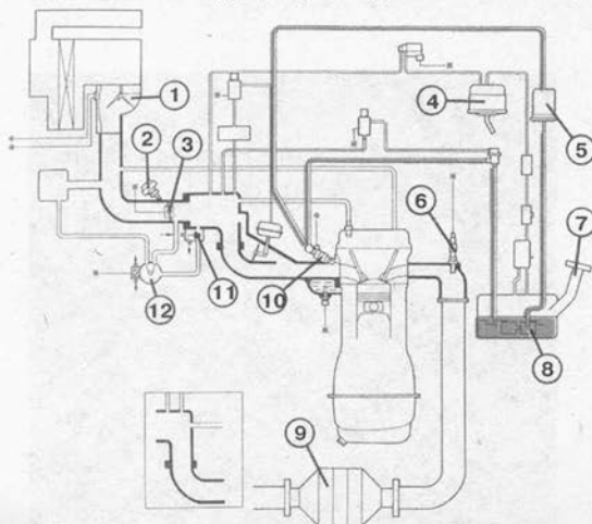
Схематическое изображение системы электронного впрыска:
