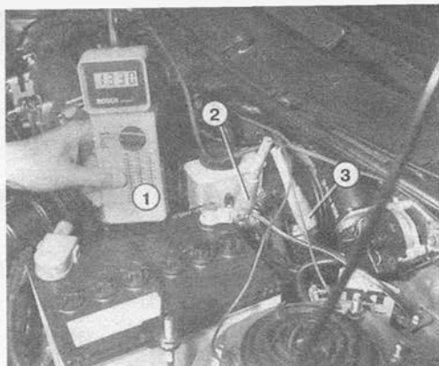
Для проверки числа оборотов к клемме «IG» диагностического разъема подключается клемма «15» (3) измерителя числа оборотов (1). Клемма «1» (2) подводится к массе батареи.
