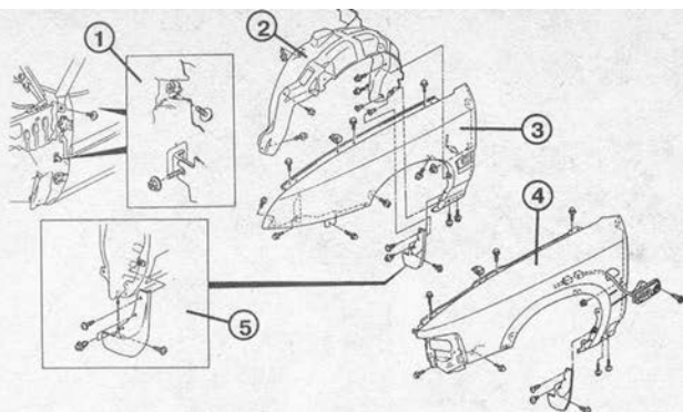
Чертеж воспроизводит вид переднего крыла. Цифрами обозначены: 1 – крепление на стойке А; 2 – свод колесной ниши; 3 – крыло F-Couré; 4 – крыло моделей с косо срезанной/ступенчатой задней частью; 5 – крепление брызговика.
