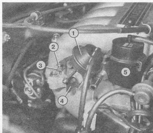
Детали управления воздухозаборными заслонками в двигателе ДОНС. Обозначены:
