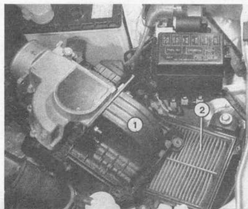
Крышка (1) кожуха воздушного фильтра снимается вместе с датчиком потока свежего воздуха. Он фиксируется на нижней части кожуха четырьмя болтами с крестообразной головкой. В нижнюю часть кожуха вкладывается патрон фильтра (2).
